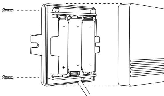
Obr. 2: Sestavení bateriového zdroje.
