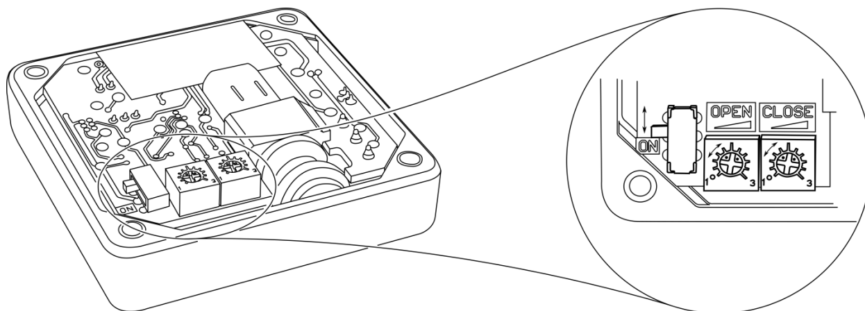
Obr. 7: Pohled na řídicí jednotku, detail na interní spínač a nastavovací potenciometry.
